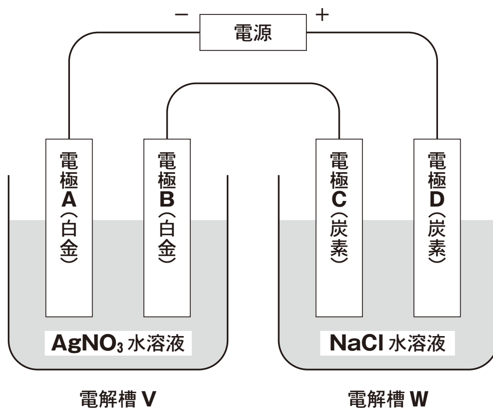
図 1 電気分解の装置
