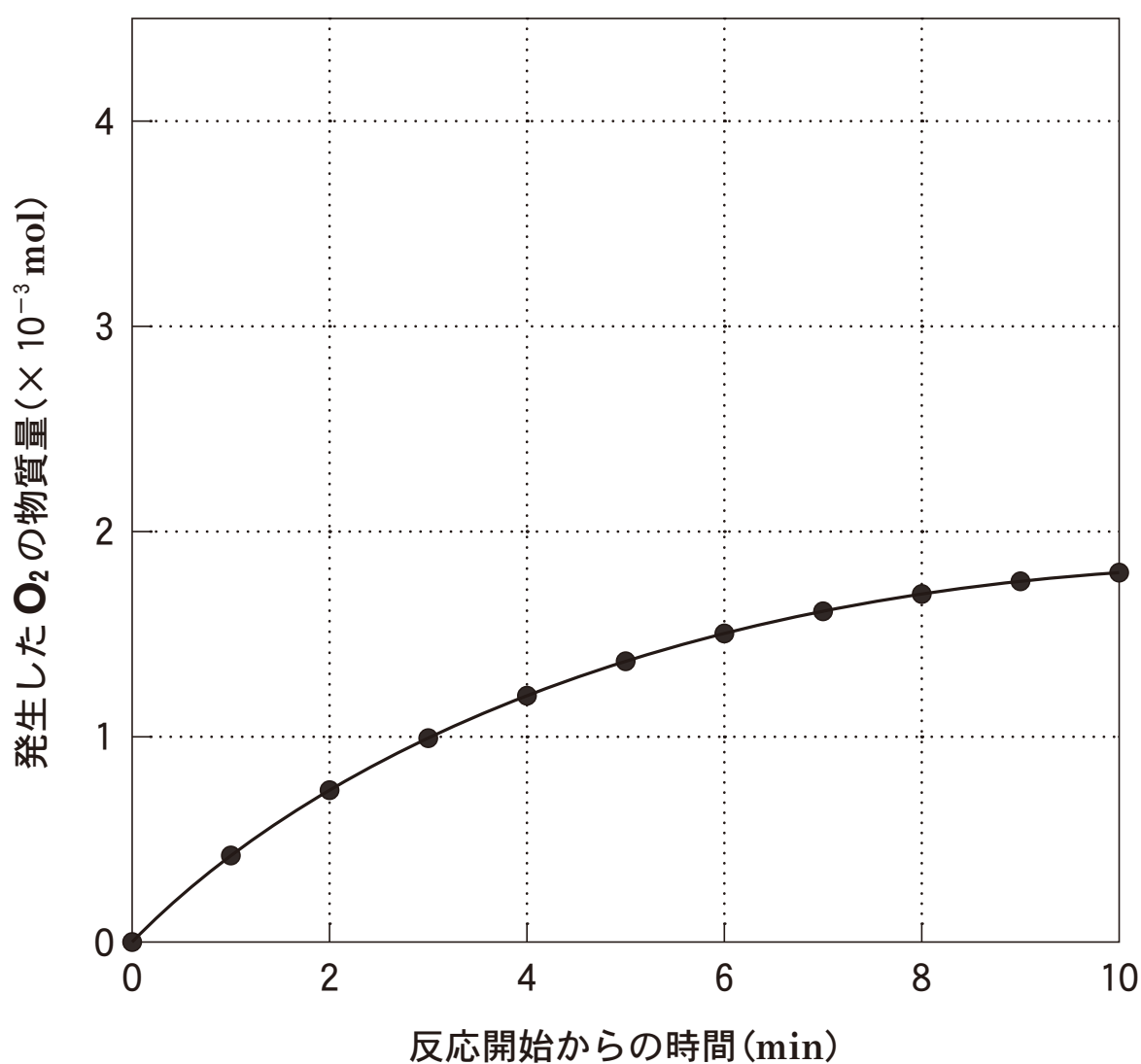
図2 反応温度 20 °C で各時間までに発生した O 2 の物質量
